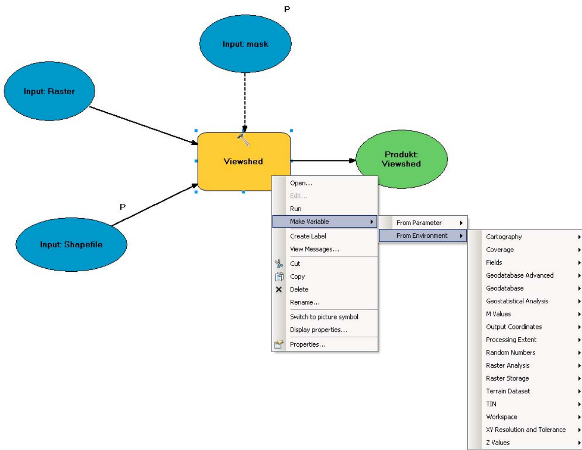
FIGUR 5: MODELBUILDER - PARAMETER
