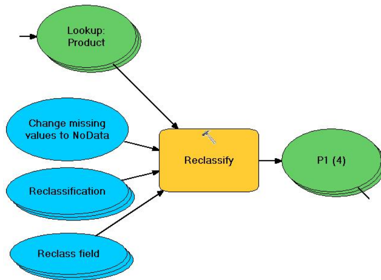
FIGUR 22: AKSEANALYSE – RECLASSIFY
