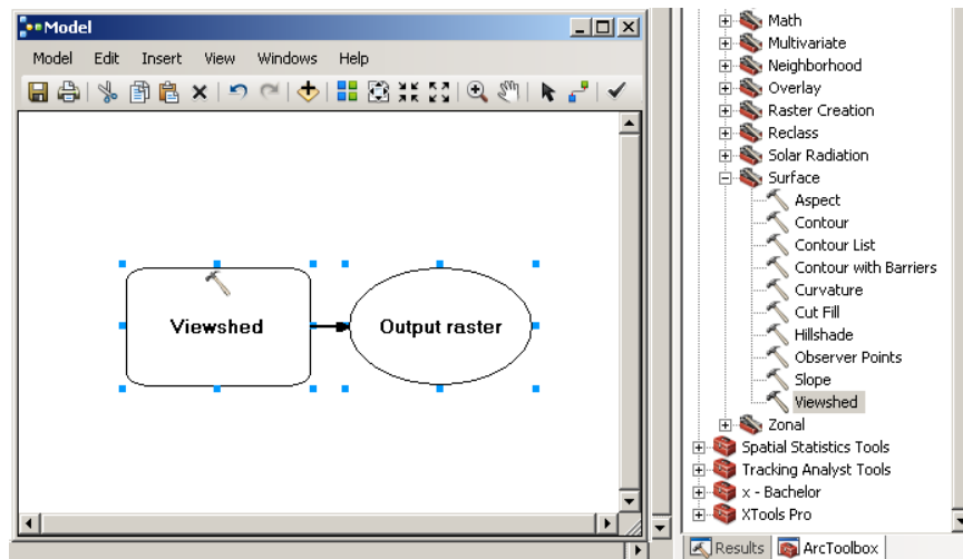
FIGUR 3: MODELBUILDER - ARBEIDSVINDU
