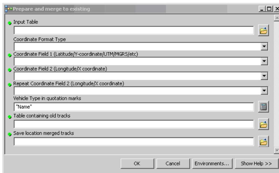
FIGUR 49: DEL 2 – DIALOGBOKS
