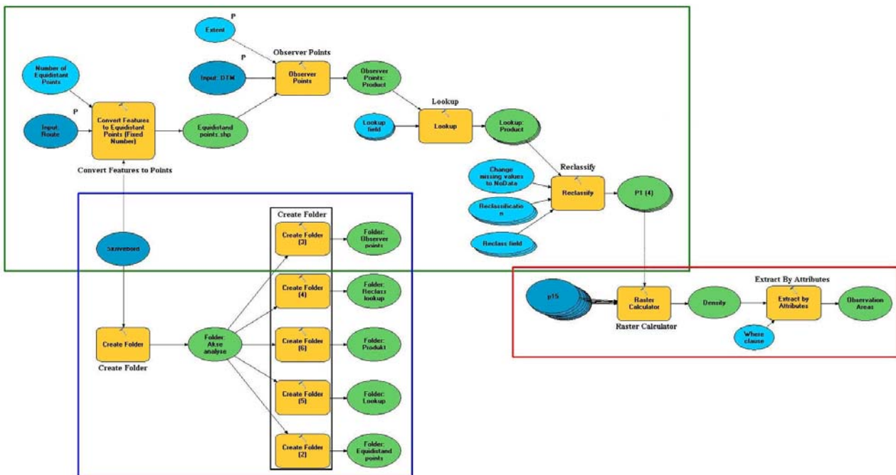
FIGUR 24: AKSEANALYSE - ORIENTERING
