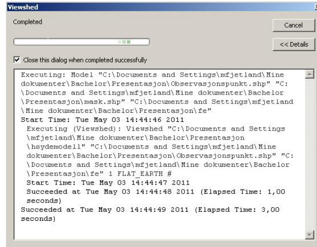
FIGUR 10: MODELBUILDER – AKTIVITETSVINDU
