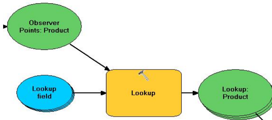
FIGUR 20: AKSEANALYSE – LOOKUP
